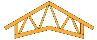
Saksiristikko
