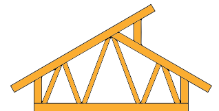
Vastaharjaristikko
