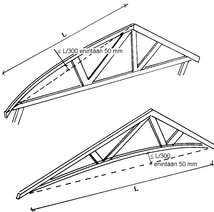
Kuva 6. Paarteiden asennustoleranssit.
